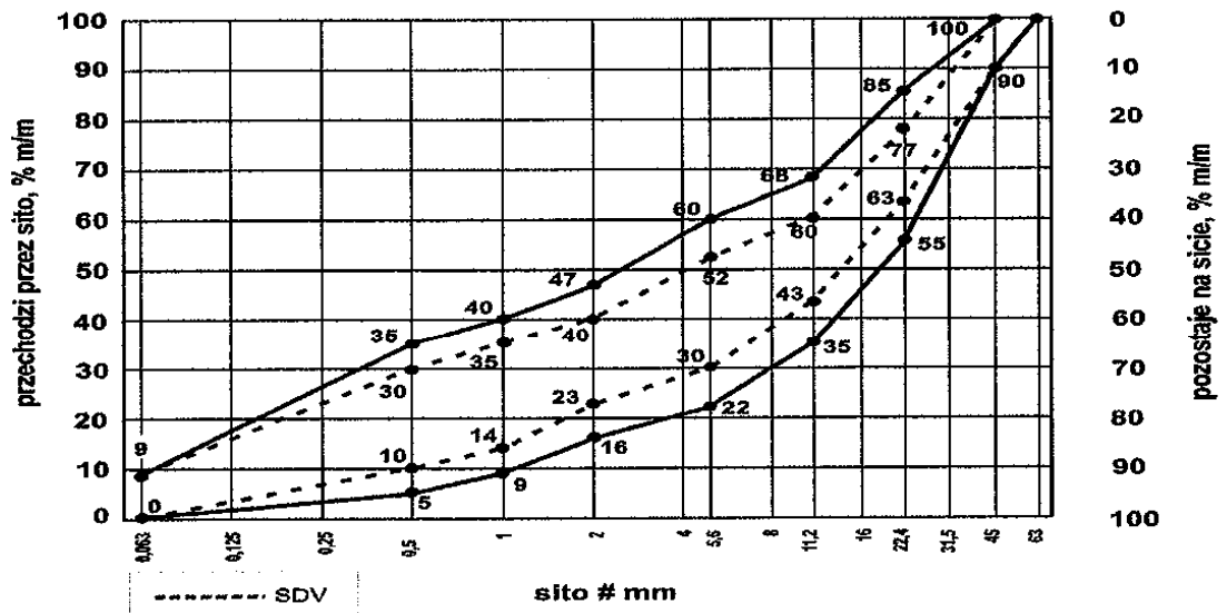
Rysunek 1. Mieszanka niezwiązana 0/31,5 do warstwy podbudowy zasadniczej
